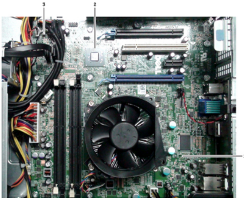
Figure 2. Carte système avec le capteur thermique et le dissipateur de chaleur retiré.
