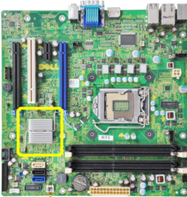
Figure 1. Version antérieure de la carte système avec le dissipateur de chaleur
